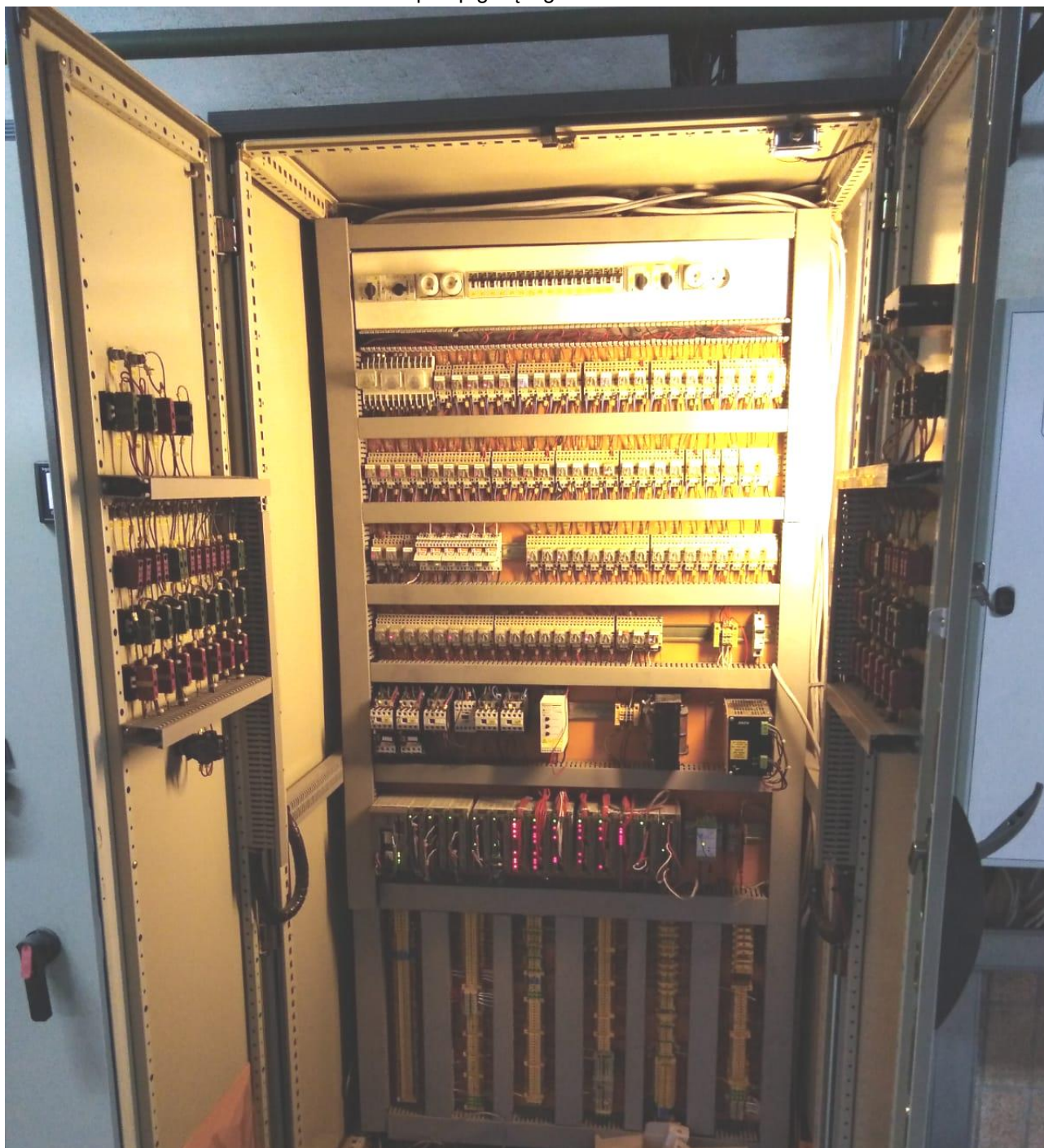
Zdjęcie nr 5 – istniejące szafy zasilająco-sterownicze. Widok wnętrza szafy sterowniczej.
