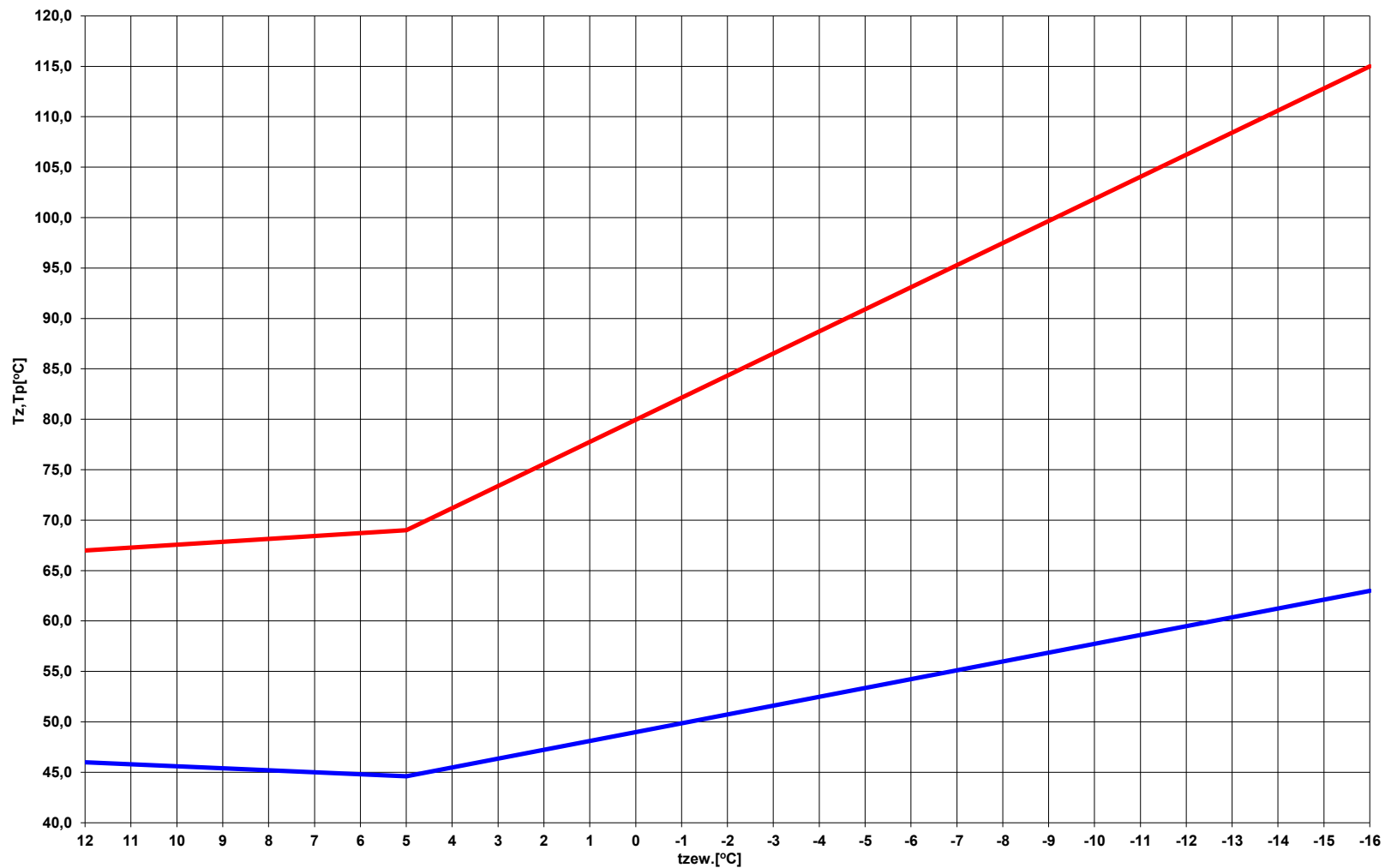
Wykres regulacyjny 115 / 63 *C dla sieci ciepłowniczej zasilanej z K-03 os. Wybickiego
